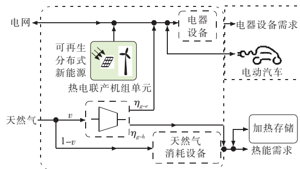
图3 住宅能源中心架构
