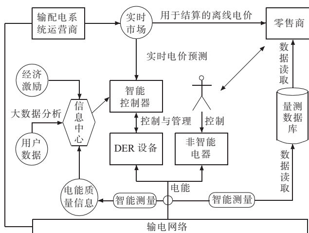
图 4 家庭用电管理应用实例
