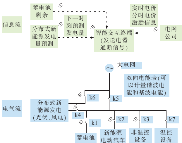
图2 家庭用电管理系统结构
