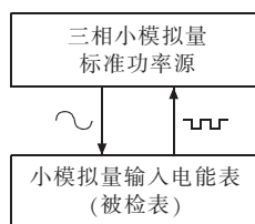
图1 小模拟量输入电能表检定示意图
