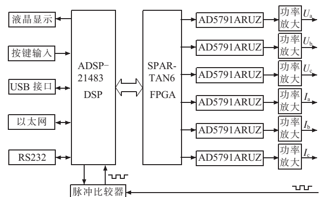
图2 三相小模拟量标准功率源硬件框图
