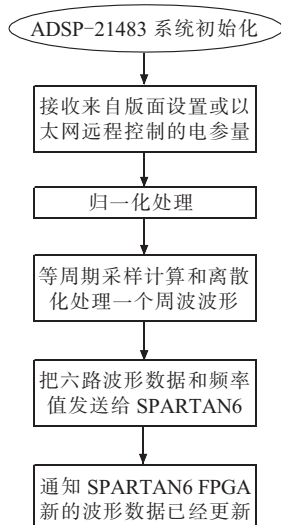
图 3 数字信号处理系统主程序框图
