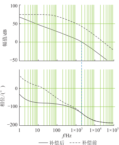
图5 DAB 输出电压环波特图
