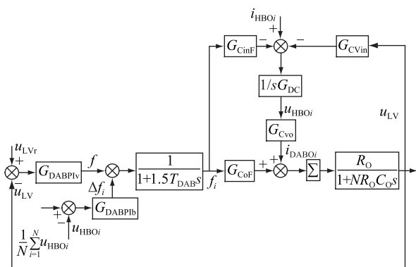
图4 DAB 控制框图
