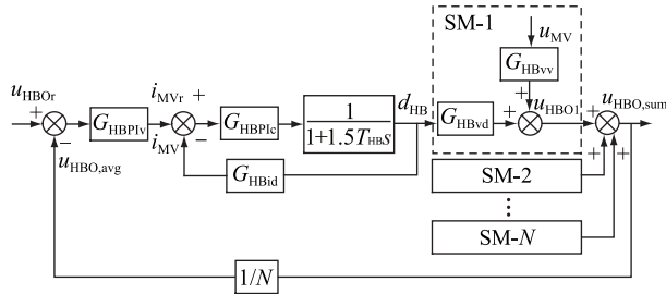
图2 HB 直流链双闭环控制框图
