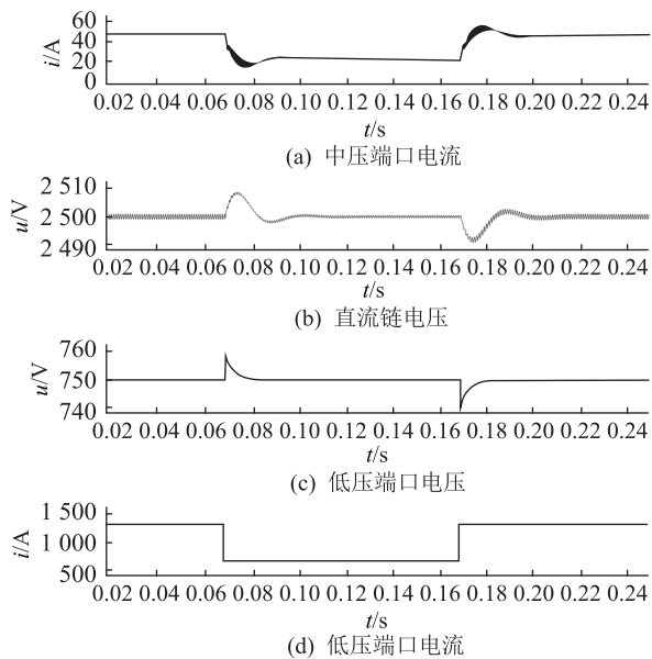
图9 负载突变响应
