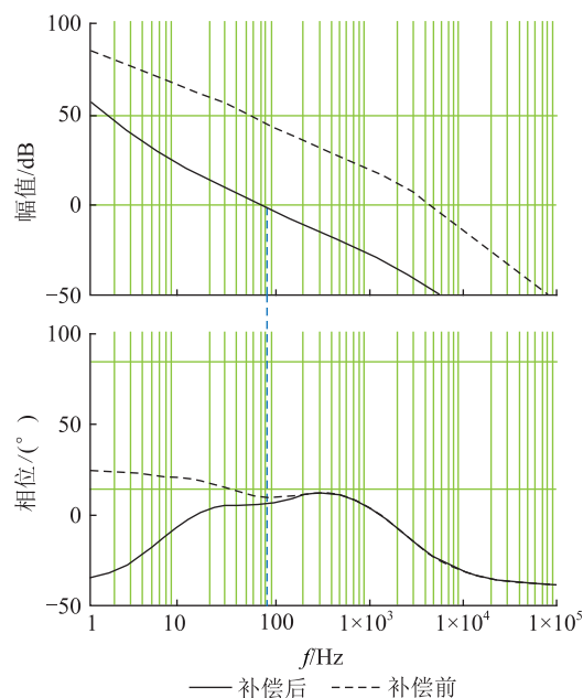
图6 DAB 均压环波特图
