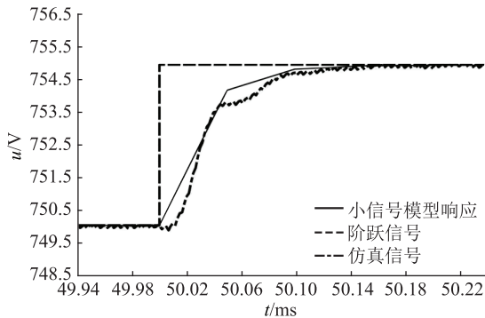
图8 DAB电路阶跃响应
