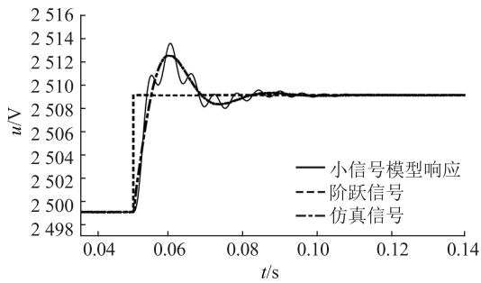
图7 HB电路阶跃响应
