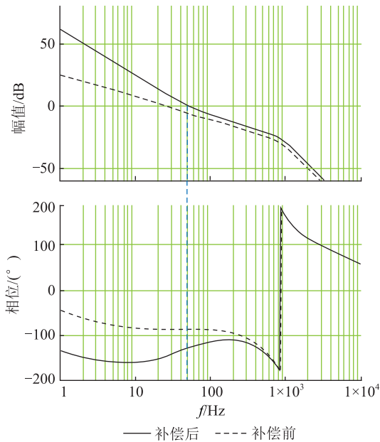
图3 HB 直流链电压环波特图
