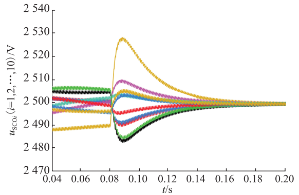
图10 直流链均压过程
